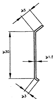
ציור 4 - מידות הפרופיל לקיבוע מכני של היריעות (המידות במילימטרים)
