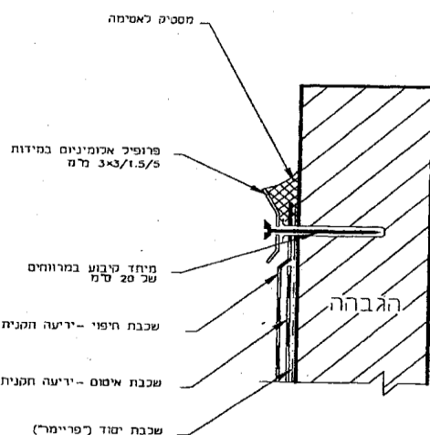
ציור 5 - דוגמה למרס קיבוע מכני
