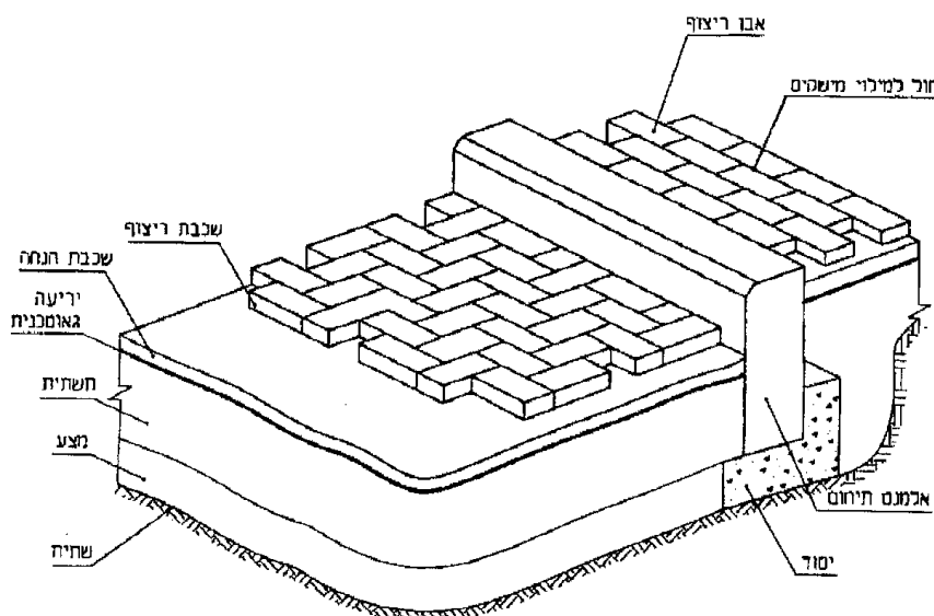
ציור 1 - מבנה טיפוסי של מיסעה מאבני ריצוף
